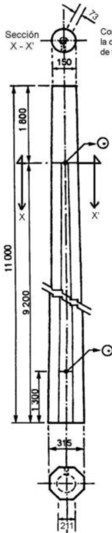
DIMENSIONES
