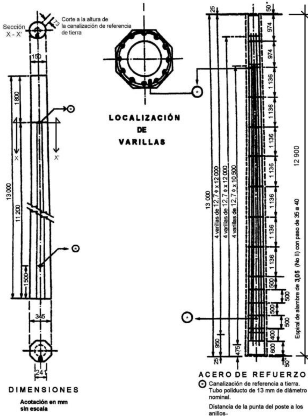
Poste PCR-13-600
